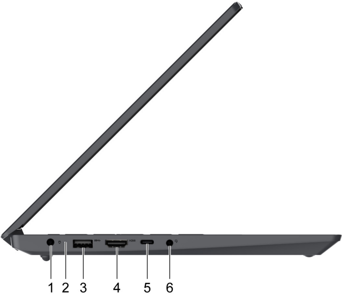
Figura 4. Vista lateral esquerda—modelos de 14 polegadas
